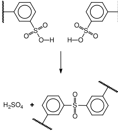
الشكل (5-6): تشبيك زمر السلفونات المتبدلية 51
