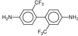
بيس (2،2'- ثنائي فلورو ميثيل ) بنزيدين
