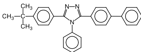
الشكل (5-9): 3-(4-بيفينيليل)-4-فينيل-5-(4-ترت-بوتيل فينيل)-4,2,1-تريازول
