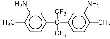
بيس (2،2'- أمينو -4- تولويل ) سداسي فلورو بروبان
