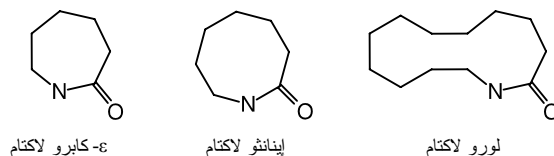
الشكل (3-12): مركبات اللاكتام المستعملة في بوليميرات بولي(فتال أميد)
