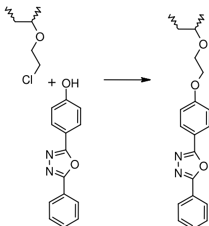
الشكل (1-6): تغيير زمر الكلور المتدلية مع 2-(4-هيدروكسي فينيل)-5-فينيل-1،3،4-أوكساديازول
