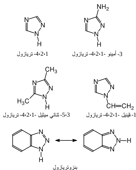
الشكل (1-9): مونوميرات تحتوي على وحدات تريازول
