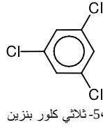
الشكل (5-2): مونوميرات مستعملة في بولي(سلفيد الفينيلين)
