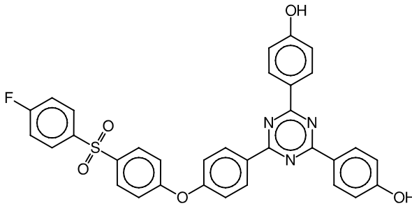
الشكل (7-8): 4,2-بيس-(4-هيدروكسي فينيل)-6-(4-4-فلوروبنزين سلفونيل)-4-بيس-(4-هيدروكسي فينيل)-1,3,5-س-تريازين
