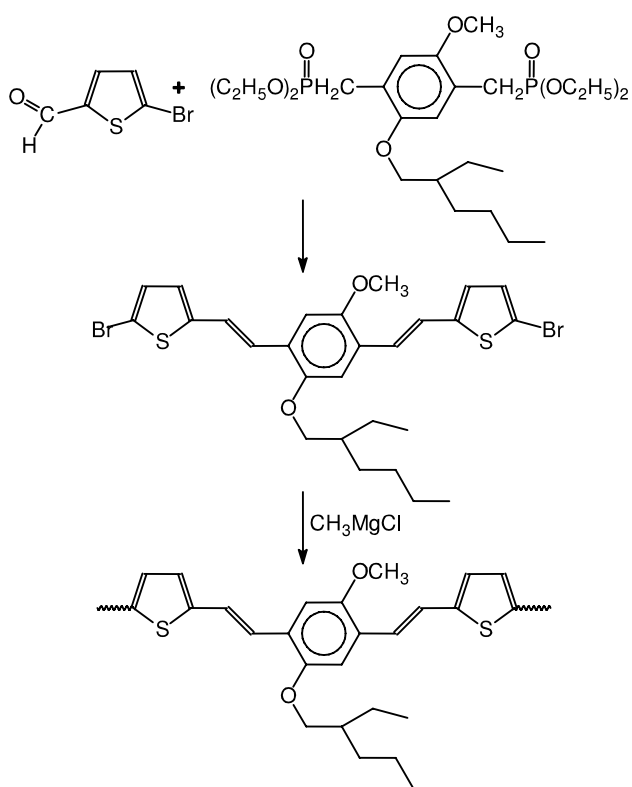
الشكل (3-6): البلمرة بمنافقة غرينيارد 13
