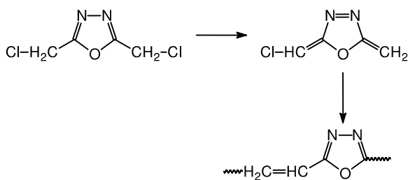
الشكل (10-7): البلمرة الآنيونية لـ 5،2-بيس - (كلوروميثيل) - 1،3،4-أوكساديازول
