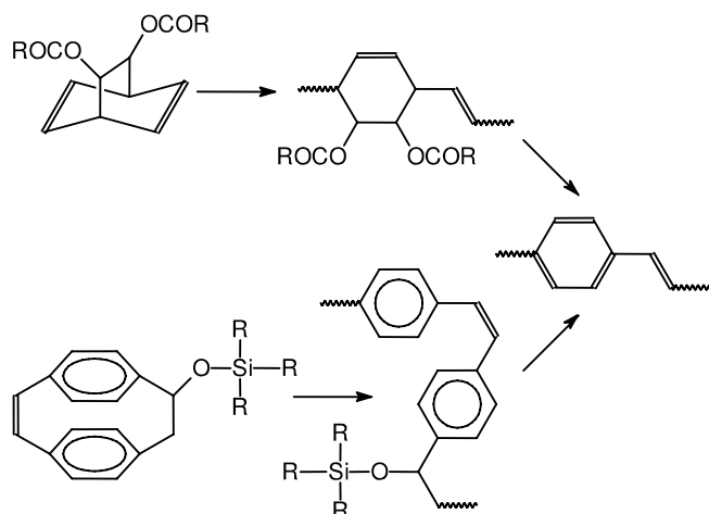
الشكل (3-5) : اصطناع PPV بواسطة البلمرة بالمناقلة الفاتحة للحلقات 12,11
