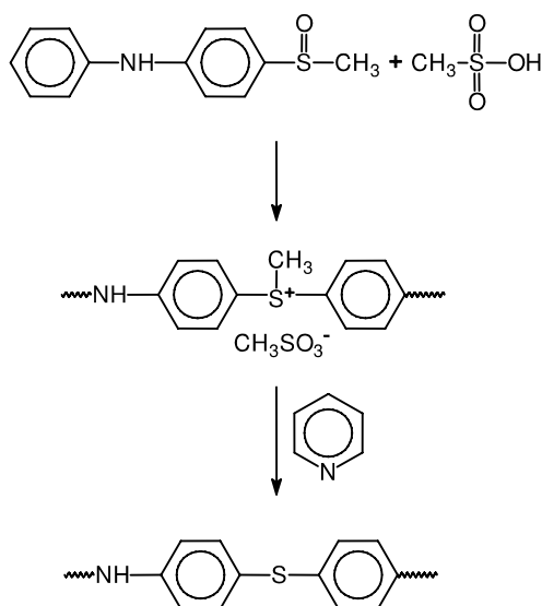
الشكل (5-6): التكايف العطري لزمرة الميثيل سُلْفونيل متبوعاً بإزالة الميثيل 47
