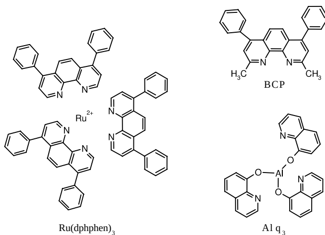
الشكل (11-1): تريس-7،4-ثنائي فينيل-10،1-فنانترولين روثينيوم (II) ، Ru(dpphen) 3 ، و 9،2-ثنائي ميثيل-7،4-ثنائي فينيل-10،1-فنانترولين، وتريس-(8-هيدروكسي كينولين)-ألومنيوم Alq_3
