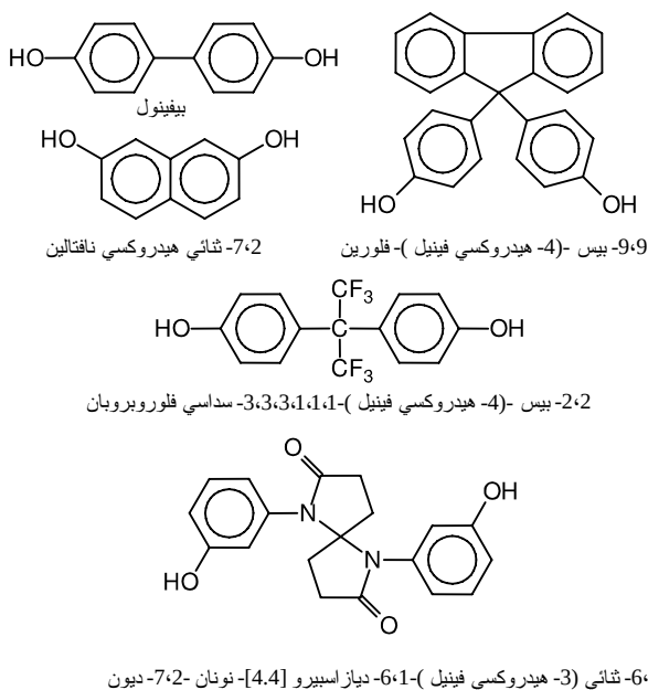
الشكل (3-8): مونوميرات الهيدروكسي في حالة بولي(أريلين إيثر نتريل)
