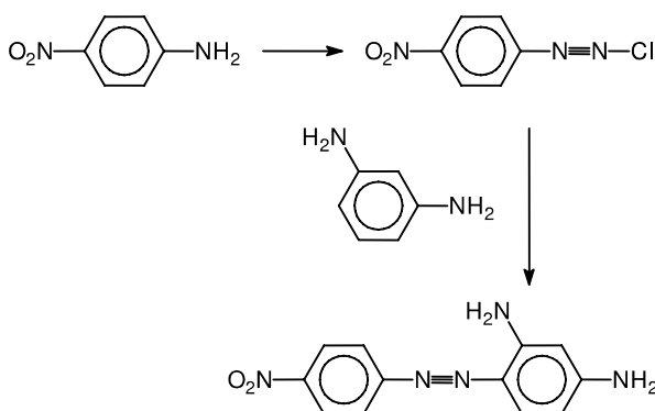
الشكل (8-14): اصطناع 4- (4'- نيترو فينيل -ثنائي آزينيل) فينيل -3،1-ثنائي أمين
