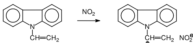
الشكل (1-7): البلمرة الكاتيونيّة لمونومير NVK
