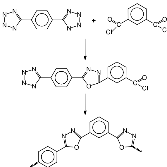
الشكل (3-10): اصطناع PODA من بيس تيترازول وكلوريد ثنائي الحمض العطري
