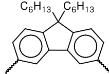
پولي(9،9-ثنائي هكسيل فلورين )
