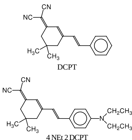
الشكل (14-1): 2-(5,5-ثنائي ميثيل-3-ستيريل-حلقي هكس-2-إينيلدين)-مالونونتريل وحوامل لون متعلّقة به 167 .
