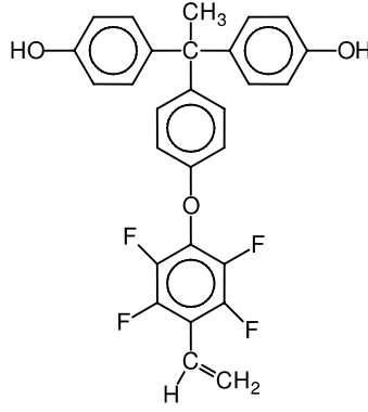
الشكل (13-7): 1،1-بيس-(4-هيدروكسي فينيل)-إيثيل-1-فينيل-2،3،5،6-رباعي
