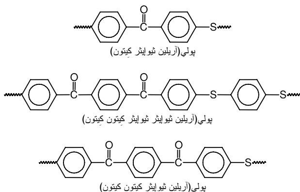
الشكل (1-5) : أنواع بولي (سلفيد الفينيلين) 4
