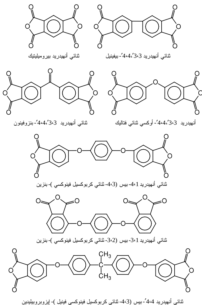
الشكل (1-15): مركبات ثنائي الأنهيدريد المستعملة في بوليميرات بولي (إيميد)
