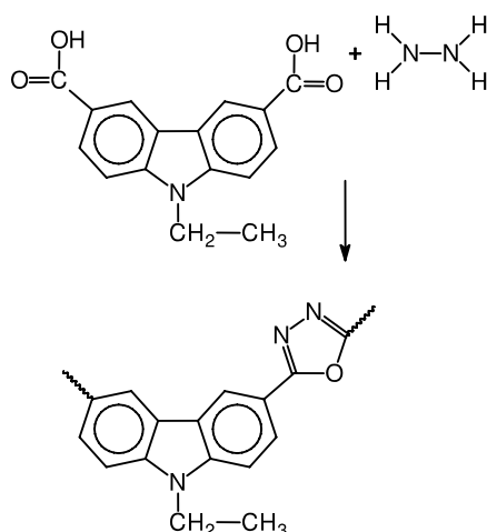
الشكل (4-10): اصطناع البوليميرات المشتركة من إيثيل كاربازول أوكساديازول 14
