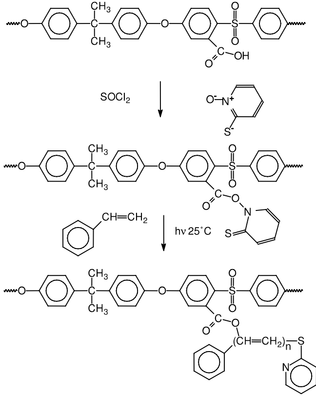
الشكل (7-9): تطعيم بوليميرات PES الموضّفة بزمركربوكسيل 55
