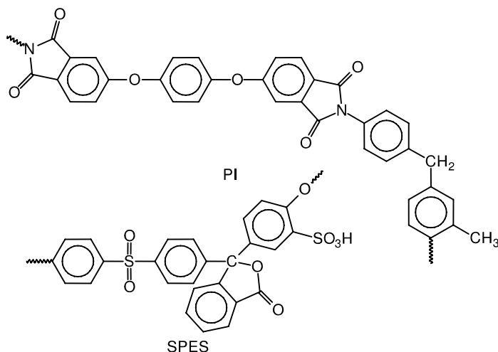
الشكل (11-7): بولي (إيميد) وبولي (إيثر سلفون) المُسلفن 81
