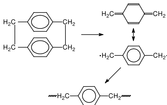
الشكل (2-3): الآلية الأساسية للبلمرة بتوضيع الأبخرة كيميائياً 32
