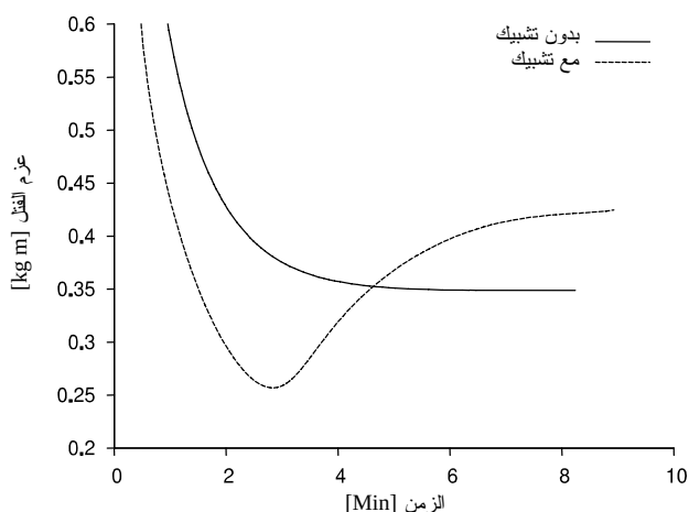
الشكل (5-4): عزم الفتل بدلالة الزمن
