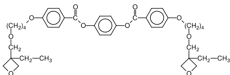
حمض بنزويك، 4-[(3-إيثيل -3-أوكسيبتانيل) ميثوكسي] بوتوكسي]-4-[[4-فينيلين إستر
