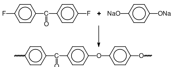
الشكل (3-6): تكاثف 4،4'-ثنائي فلوروثنائي فينيل كيتون مع هيدروكينون
