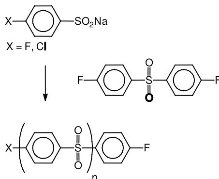
الشكل (3-7): تكاثف 4-هالو بنزين سلفينات المحفز بـ 4,4'-ثنائي فلورو ثنائي فينيل سلفون
