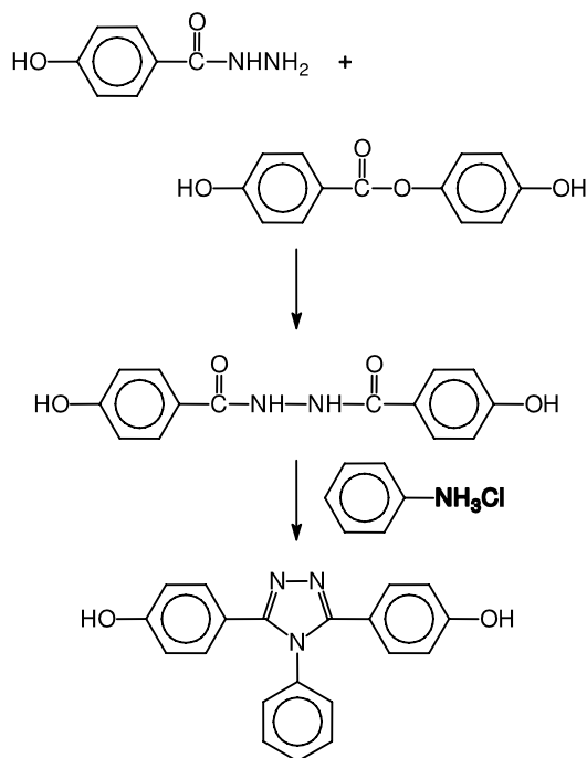
الشكل (2-9): اصطناع مونوميرات ثنائي (هيدروكسي فينيل) - 4،2،1-تريازول 2
