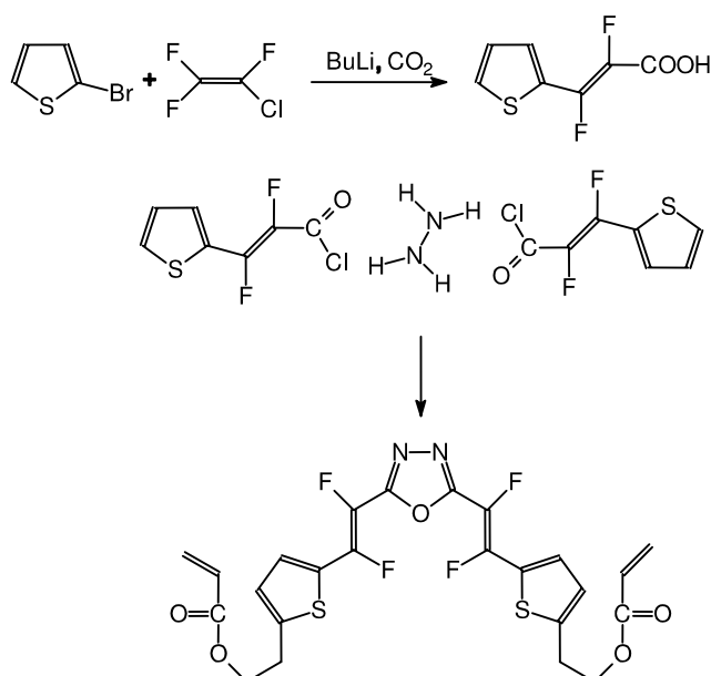
الشكل (2-10): اصطناع مونومير أوكساديازول قابل للتشبيك التسالبي 7
