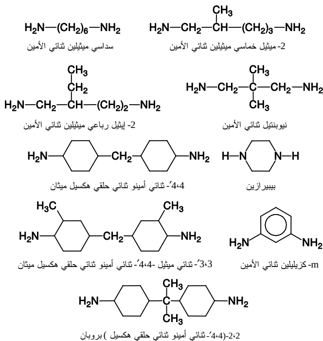
الشكل (2-12): ثنائيات الأمين المستعملة في بوليميرات بولي(فتال أميد)
