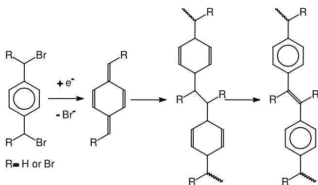
الشكل (3-7): اصطناع بوليمير (p-فينيلين فينيلين) بالبلمرة الكهربائية
