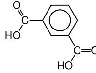
حمض إيزوفتاليك
