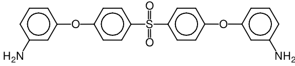
بيس (4-3- أمينو فينوكسي ) فينيل [سلفون
