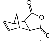
أنهيدريد ناديك
