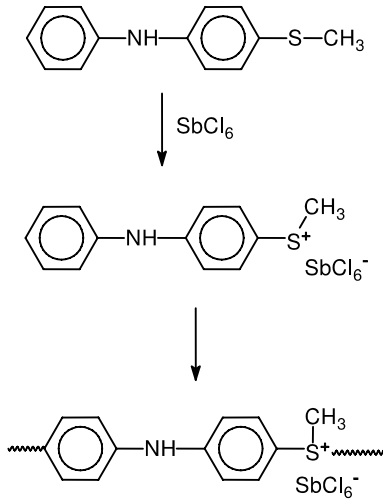
الشكل (5-7): تكاثف بتكاثف ميثيل-(4- أنيلينوفينيل) سلفيد مع خماسي كلور الأنتيمون
