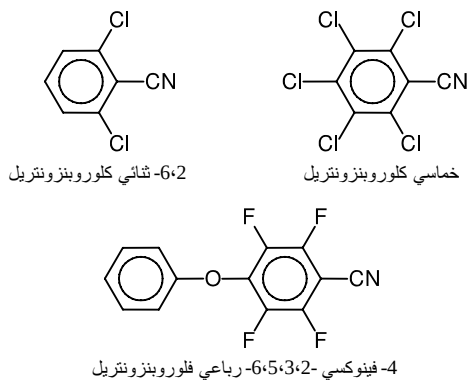
الشكل (2-8): مونوميرات النتريل في حالة بولي(أريلين إيثر نتريل)
