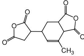
ثنائي أنهيديد 5- (5،2- ثنائي أوكسو رباعي هيدرو فوريل )-(3- ميثيل -3- حلقي هكسين -2،1- ثنائي كربوكسيليك
