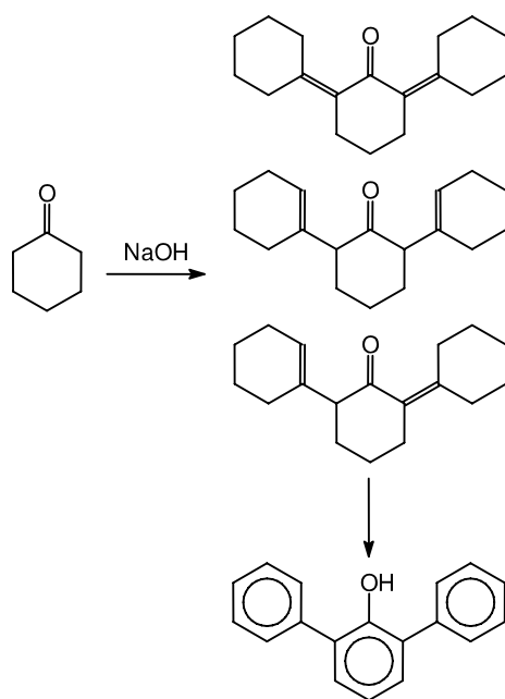
الشكل (4-2) : اصطناع 6،2-ثنائي ميثيل فينول من الكزانول الحلقي مروراً بثلاثة إيزوميرات وسيطة 15
