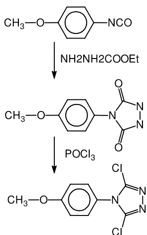
الشكل (4-9): اصطناع 5،3-ثنائي كلورو -4- (4-ميثوكسي فينيل) -4H-2،1-تريازول 11
