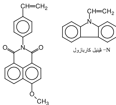
الشكل (1-9): مونوميرات مشتركة للمواد الناقلة للشحنة 58
