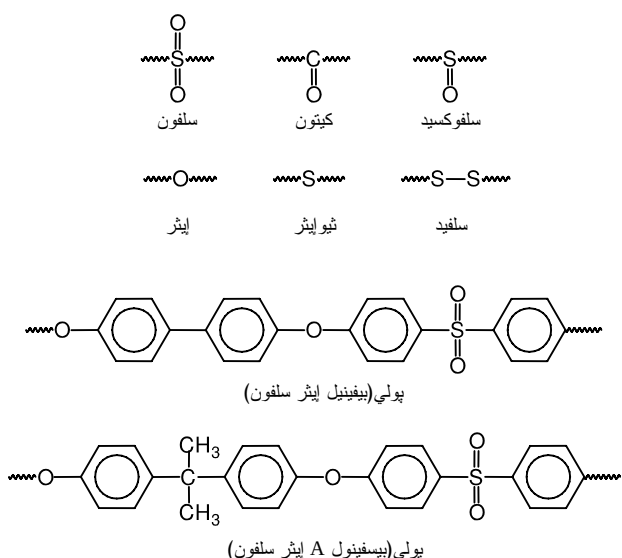
الشكل (1-7): الزمر الوظيفية وكتل بناء أنماط من بولي(اثير سلفون)
