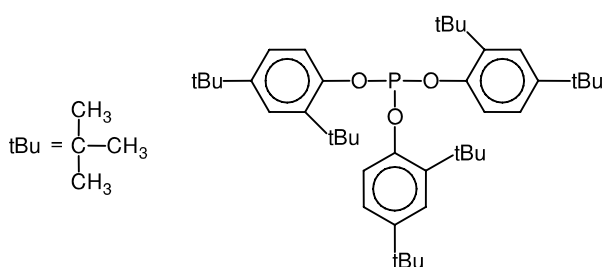
تريس (4،2- ثنائي- تريت- بوتيل فينيل) فوسفيت
