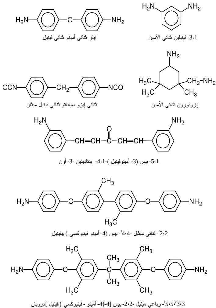
الشكل (2-14): ثنائيات الأمين وثنائيات الإيزوسيانات المستعملة في حالة البولي (أميد إيميد)
