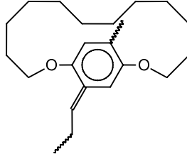
الشكل (3-15): الوحدات المتكررة في بوليمير (2،15-ثنائي أوكسابيسيكلو (2.2،14) إيكوزا - 16،19،20،17- تريين - 17،19- إيلين فينيلين ) (BDA-PPV) 29
