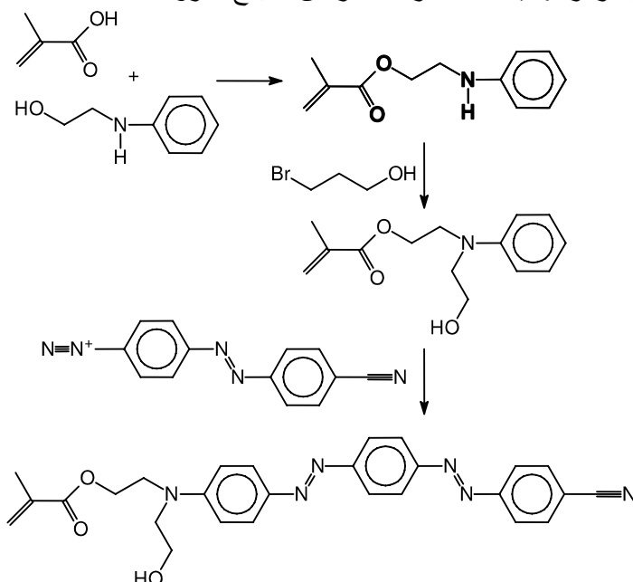
الشكل (7-16): اصطناع ميتاكريلات محتو على آزوبنزين 59
