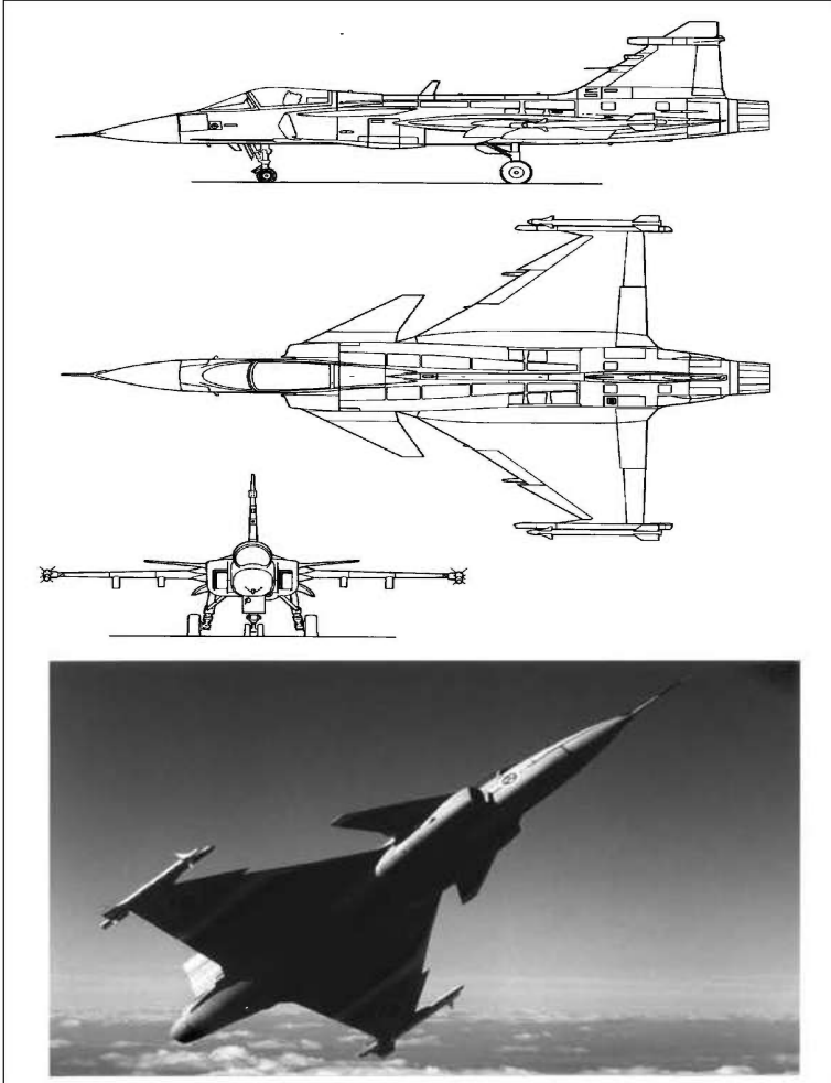
الشكل 17 - 3 طائرة كنار حديثة، ساب جاز 39 غريبن (SAAB JAS 39 Gripen). (من: Jane's All the World's Aircraft, 1987-1988).
