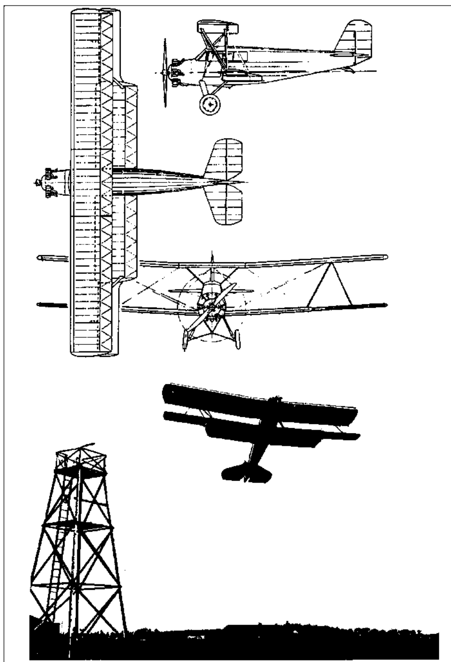
الشكل 15 - الطائرة كورنيس تناجر، بقلابات وقدرات على كامل باع الجناح، قدمت عرضاً لتسلق حاد فوق حاجز ارتفاعه 35 قدماً، وفازت هذه الطائرة بمنافسة الطائرة الآمنة لكوغنهايم (من : Pendray, The Guggenheim Medalists, 1929-1963 ).
