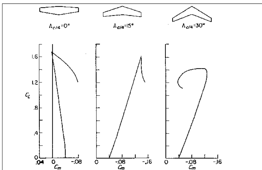
الشكل 11 - 8 تأثير التراجع للخلف في توقف معامل عزم التسلق/ الانحدار عند الانهيار. الأجنحة المستقيمة والمترجمة بمقدار 15 درجة تكون مستقرة ما بعد الانهيار؛ ويكون الجناح المترجع بزاوية 30 درجة غير مستقر (أنف للأعلى). (من : Furlong and McHugh, 1957, NACA Rept. 1339).
