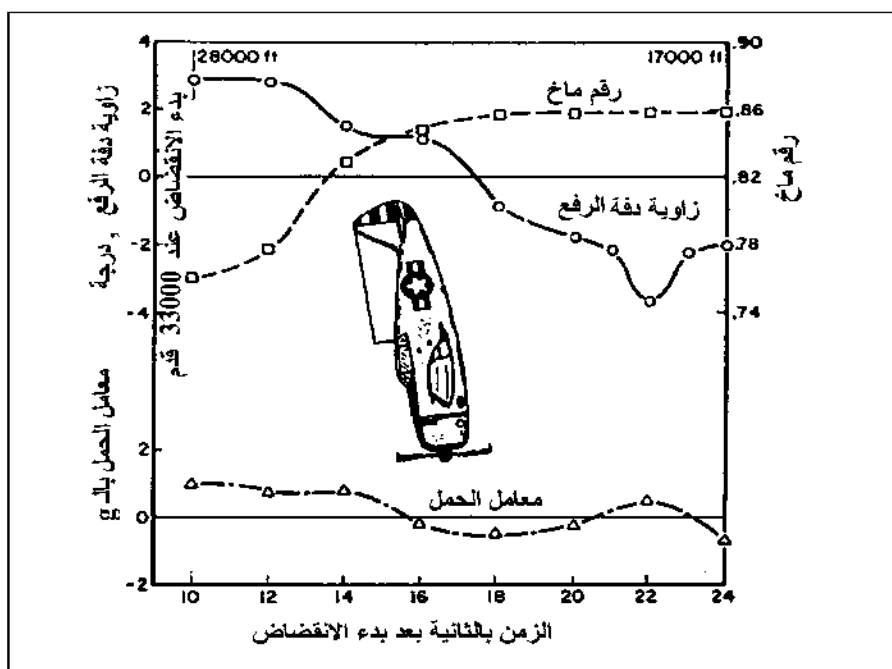
الشكل 11 - 4 إخفاق الطائرة ثونديربولت في التجاوب مع 4 درجات دقة رفع إلى الأعلى في انقضااض عند رقم ماخ 0.86 . (من : Perkins, Journal of Aircraft , July-August 1970).
