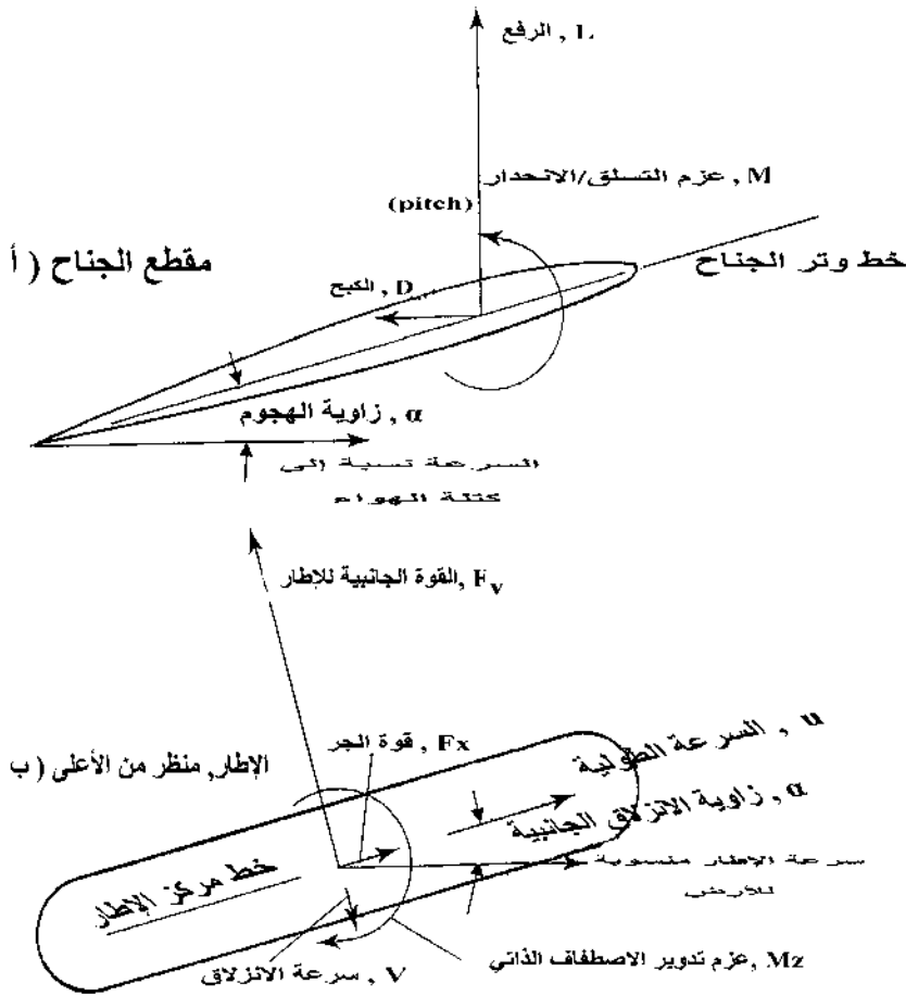
الشكل 14 - 8 العزوم والقوى الفاعلة في مقاطع الجناح (أ) وفي دوران الإطارات (ب) (من: (Abzug, 1999).
