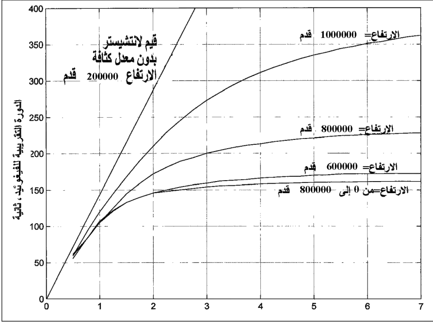
الشكل 11 - 17 تغيرات تقريب دور الحركة الاهتزازية البطيئة (الفيغوييد) مع الارتفاع ورقم ماخ، متضمنة معدل الكثافة مع تأثيرات الارتفاع.
