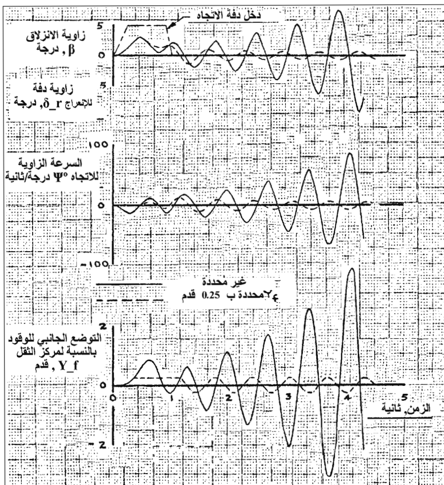
الشكل 14 - 1 التأثير المحسوب لخضضة خزان الوقود في الطائرة دوغلاس سكايبوك A-4 قبل تركيب المصد في الخزان. تترافق حركة الوقود مع نمط حركة الفيغويثيد. وعندما تتحدد حركة الوقود بجوانب أو جدران الخزان (المنحني المنقط) تنتج حركة «افعوانية» محدودة التمدج (من: Abzug, Douglas Report. ES 2955, 1959).
