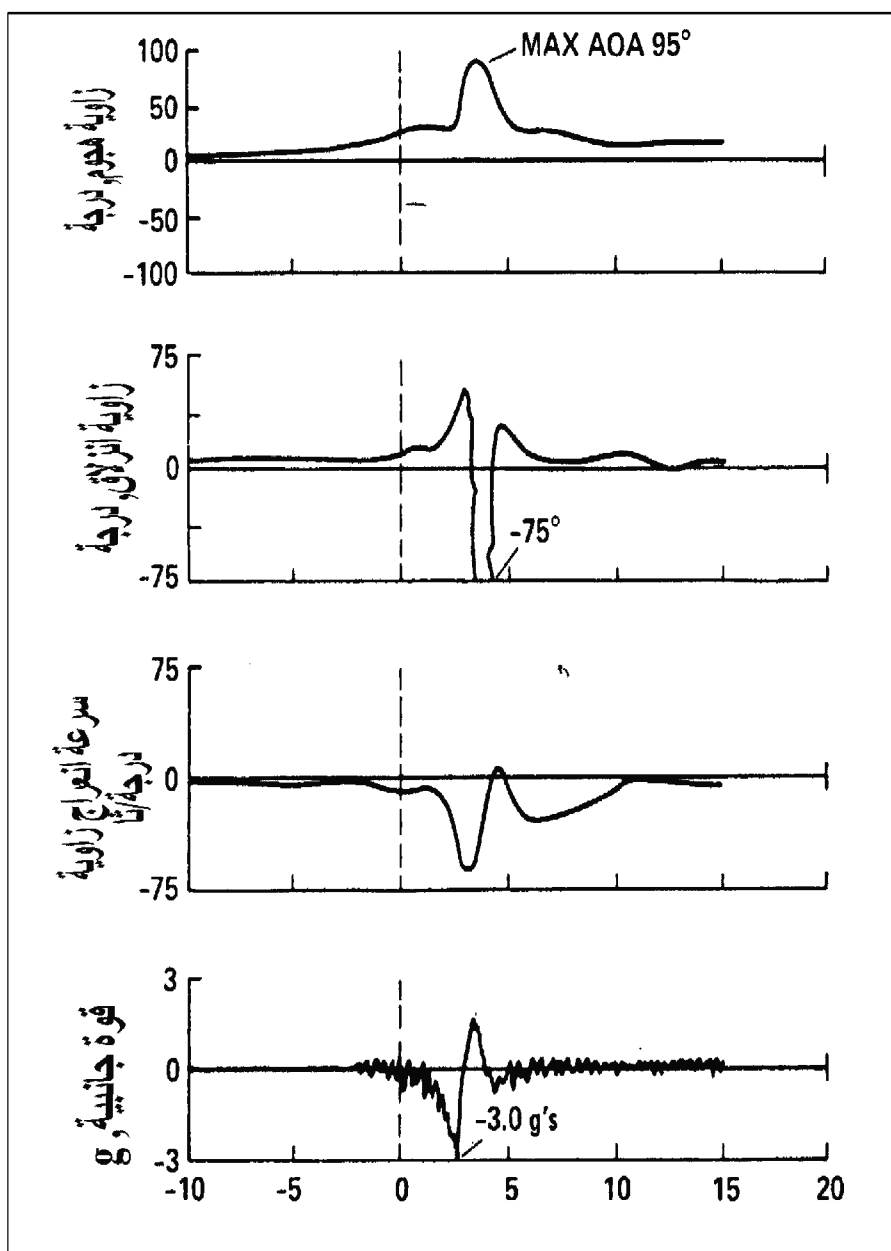
الشكل 9 - 13 مغادرة الانعراج على الحدود الصوتية التي تم الحصول عليها مع الطائرة ماك دونيل دوغلاس F/A-18A باستخدام التحكيمات ما قبل الحركة الحلزونية، أو دفات دحرجة ودفة اتجاه مضادة، مع الدحرجة بزاوية هجوم وسطية (من : Anderson, Enevoldson, and Nguyen, AGARD CP-347, 1983).
