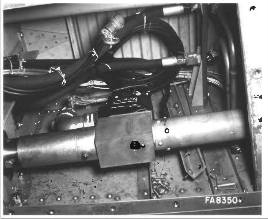
الشكل 20 - 1 مشغل من النوع المتسلسل (مخدم بوابة طرح الفضلات) المستخدم في الطائرة بوينغ XB-47 ستراتوجيت لدفع قضيب دفة التوجيه، وتأمين تخميد بالانمرج (من : White, 1950 Journal of the Aeronautical Sciences (Honeywell)).
