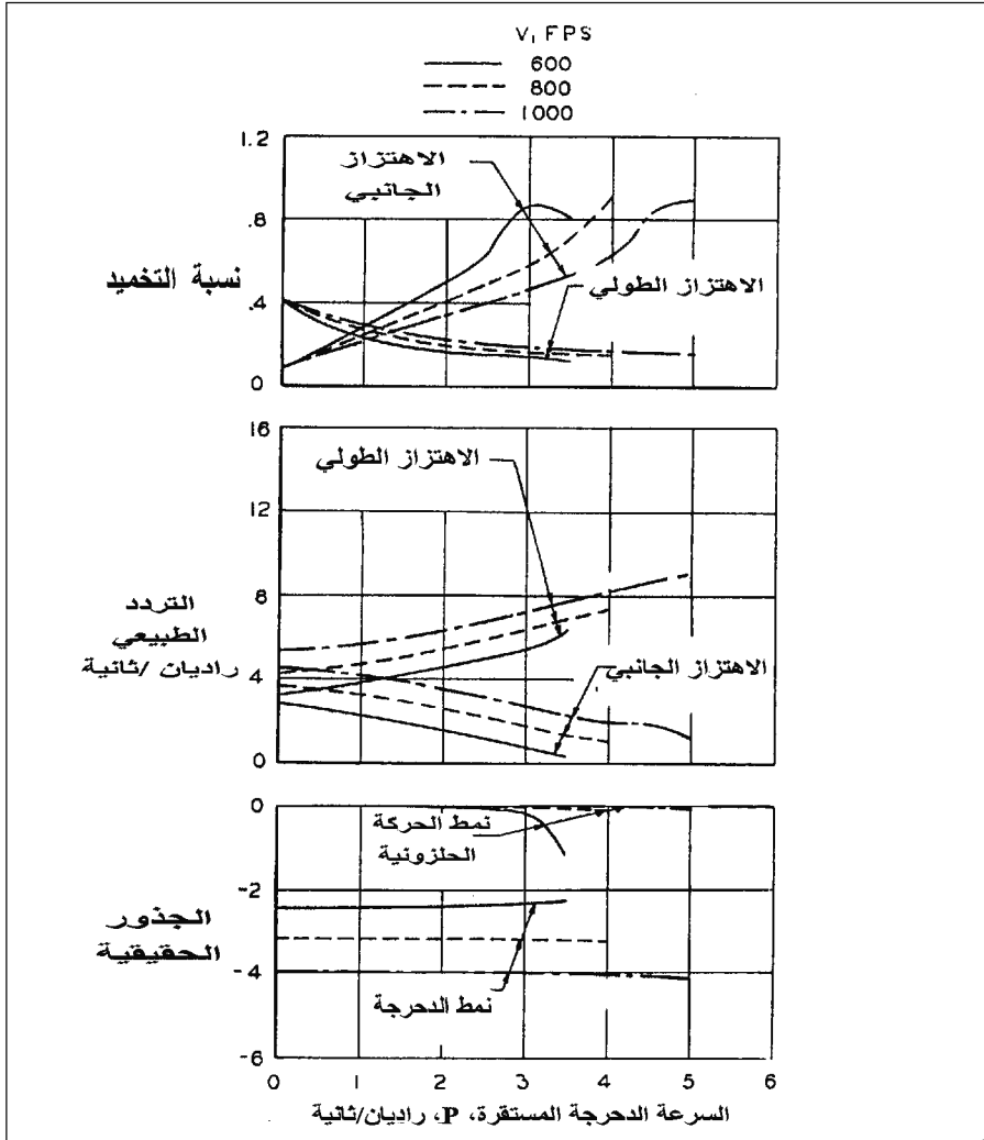
الشكل 8-6 تأثير الدحرجة الوئيدة (steady rolling) على الاضطراب الصغير لأنماط حركة الطائرة دوغلاس F4D-1. أخذت حامد الحركة الاهتزازية الطولية السريعة عند سرعات دحرجة زاوية عالية نصف قيمته (من: Abzug, Journal of the Aeronautical Sciences , November 1954).
