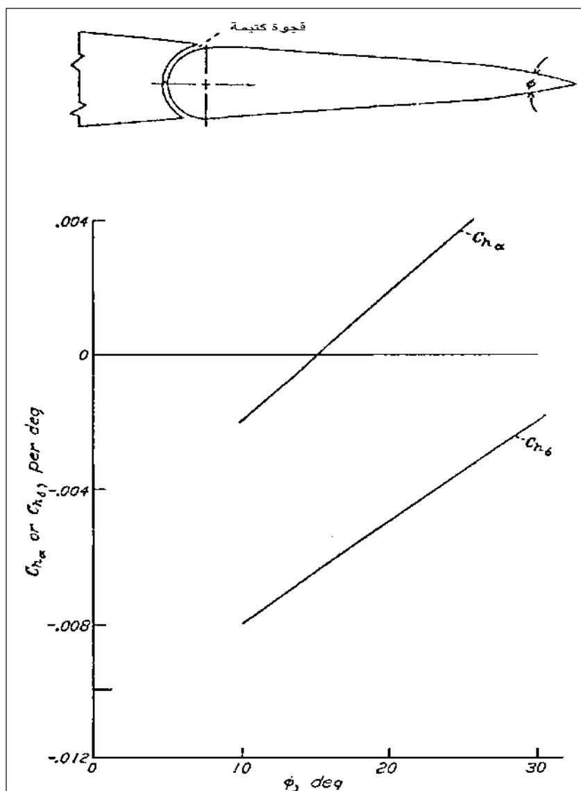
الشكل 5-8 - تغير معيار عزم المفصل التالي مع زاوية الشد \phi لسطح تحكم مشدوف. (من: Phillips, NACA Rep. 927, 1948).
