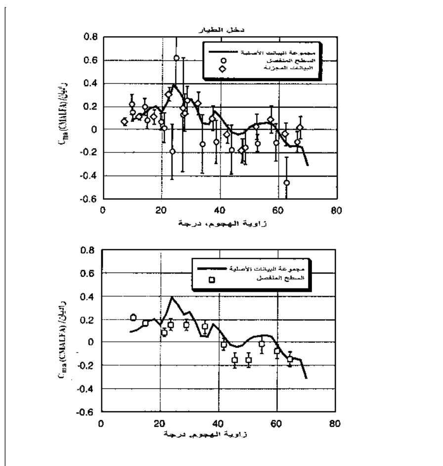
الشكل 14 - 17 تحسين التعرف بـ C_{ma} على الطائرة X-31A مع مدخلات (inputs) سطح تحكم منفصل (غير مغلق بحلقة تحكم). (من : Weisc, Journal of Aircraft , 1996).
