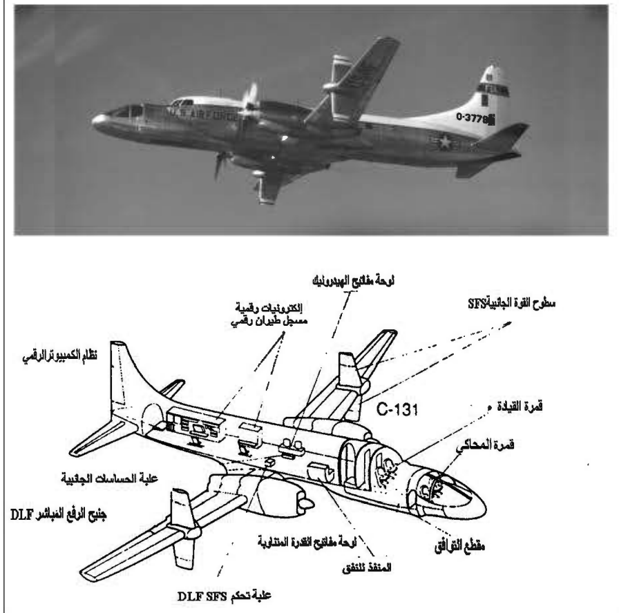
الشكل 3- 12 الطائرة متغيرة الاستقرار TIFS (محاكي طيران كامل)، بنتها غالسبان عن طائرة سلاح الجو كونفير C-113B. تستطيع الطائرة توليد رفع مباشر وقوة جانبية (من : Phillips, Journal of Guidance, Control, and Dynamics , July-August 1989).
