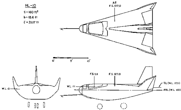
الشكل 14 - 19 المساقط الثلاثة للجسم الرافع ناسا/ نورثروب HL-10 (من : Heffley and Jewell, NASA CR-2144, 1972).
