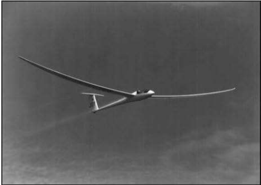
الشكل 19 - 7 تقوس الأجنحة المرننة إلى أعلى للطائرة الشراعية عالية الأداء المصنعة من الألياف الزجاجية. يهيف التقوس إلى فعالية زاويتها الثنائية (Photo Steve Hines).
