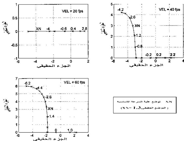
الشكل 14 - 9 القيم الخاصة للدرج الأرضي للطائرة سيسنا 182 عند 3 سرعات (Abzug, 1999).
