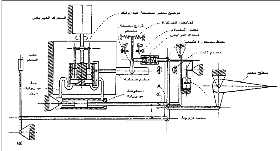
الشكل 5 - 16 أول نظام تحكم تجريبي معزز هيدروليكياً ركبته NACA على دفة رفع الطائرة بوينغ B-29. تضبط نسبة التعزيز l/d من خلال ضبط موضع النقطة (a). (من : Mathews, Talmage and Whitten, NACA Rep. 1076, 1952).
