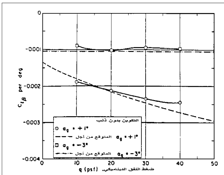
الشكل 19-8 تأثير الضغط الديناميكي في أثر الزاوية الشنائية للطائرة دوغلاس XA3D-1، عند زاويتي هجوم. يكون رفع الجناح قريباً من الصفر عند زاوية هجوم للجسم تساوي 3 درجة، وهنا انحناء قليل للجناح وتغير في أثر الزاوية الشنائية (من: Rodden, AGARD Report 725, 1989).
