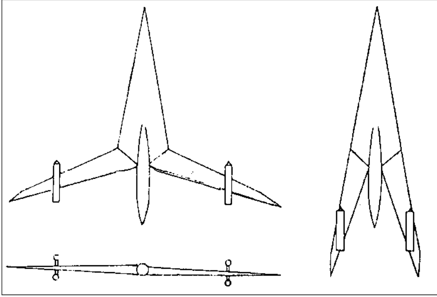
الشكل 16 - 6 تصميم فيكيرز - ارمسترونغ (Vickers-Armstrong) «السنونو» بتراجع متغير، اختبرت في غير لانغلي في الناسا ووجدت أنها غير مستقرة طولياً عندما تكون الأجنحة غير متراجعة (من: Polhamus and Toll, NASA TM 83121, 1981).
