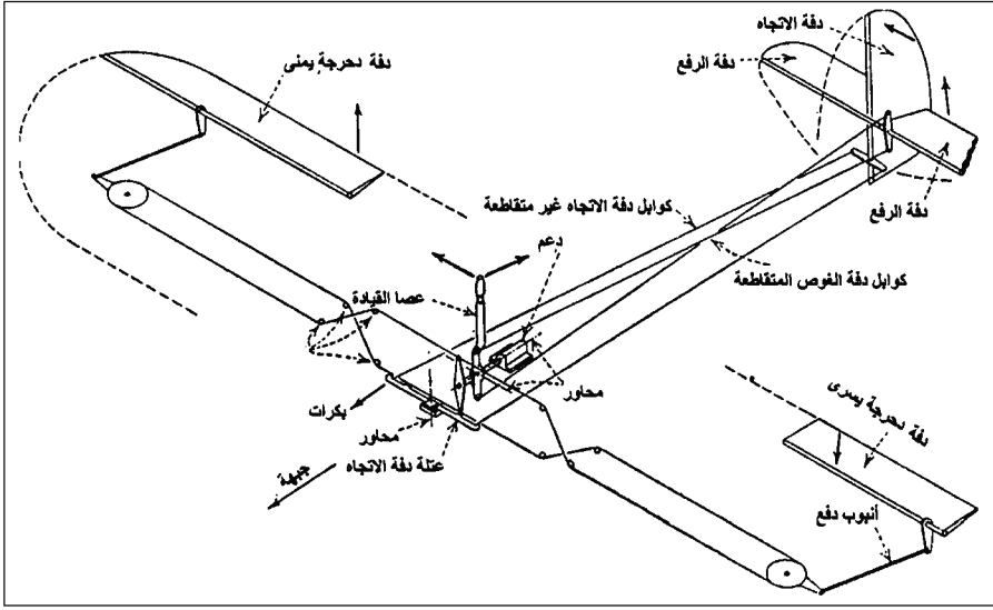
الشكل 1 - 3 رسم تخطيطي لنظام تحكم بسيط بطائرة. يتم التحكم بسطوح التحكم من خلال تحريك العصا وقضيب دفة الاتجاه وفق مؤشرات الأسهم. (من : Chatfield, Taylor, and Ober, The Airplane and its Engine , McGraw-Hill, 1936).
