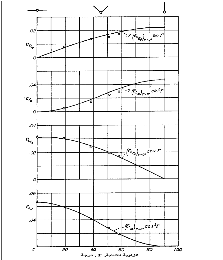
الشكل 14 - 12 التحقق التجريبي (الدوائر الصغيرة) لنظرية بورسر/ كامبيل في الذنب V. رسمت مساهمات معزولة لاستقرار وتحكم الذنب مقابل زاوية الذنب الشنائية (من: Purser and Campbell, NACA Rept. 823, 1945).
