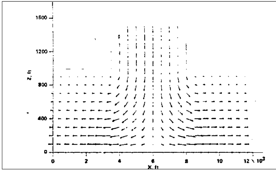
الشكل 18 - 11 المقطع العمودي العرضي في نموذج برية للدفق السفلي (Bray model of down - burst). طول الأسهم متناسبة مع سرعة جريان الهواء (من : Bray, NASA TM 85969, 1984).
