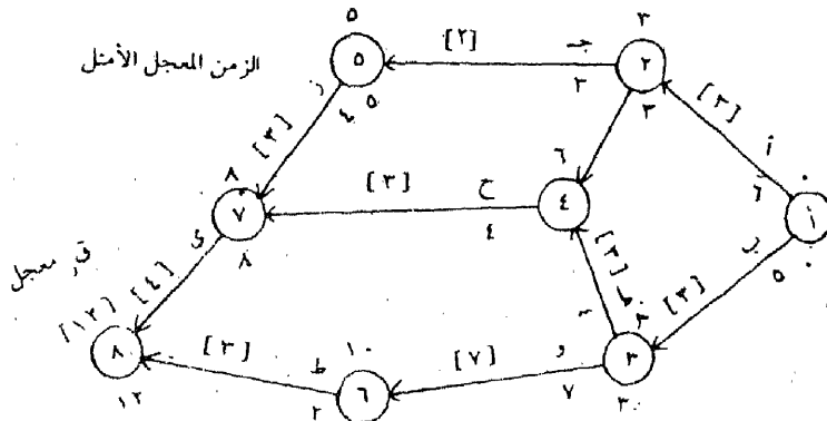
شكل (١١/٩) خريطة التتابع الفني مع التعجيل الأمثل في وقت ق، معجل تنفيذ معجل قدره ١٢ أسبوعاً.
