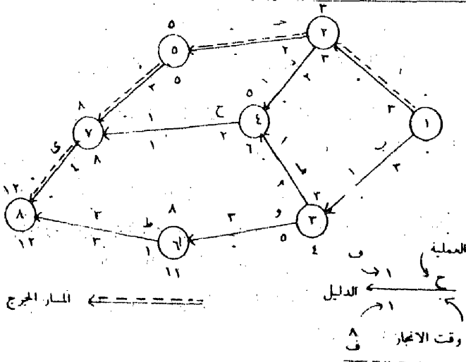
شكل ( ٩/١٠ ) خريطة التتابع العمي في ظل رسم الإنجاز المعجل مع الفائض الكلي والفائض الحر للعمليات
