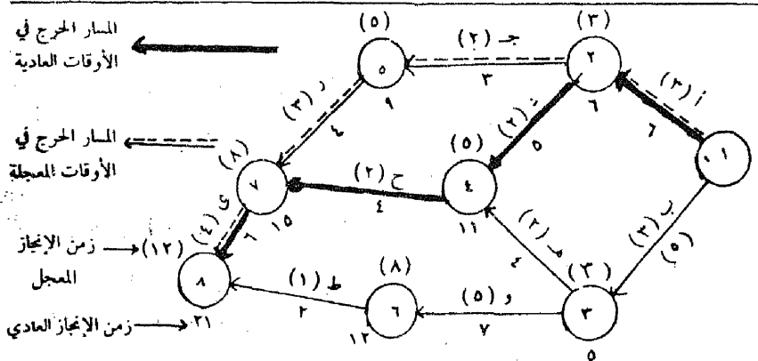
شكل (٧/٩٠) خريطة التتابع الفني وزمن الإنجاز العادي والمعجل للأنشطة
