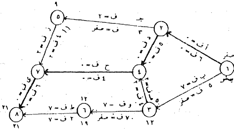
شكل ( ٩/١٠ ) خريطة التتابع العمي في ظل رسم الإنجاز المعجل مع الفائض الكلي والفائض الحر للعمليات
