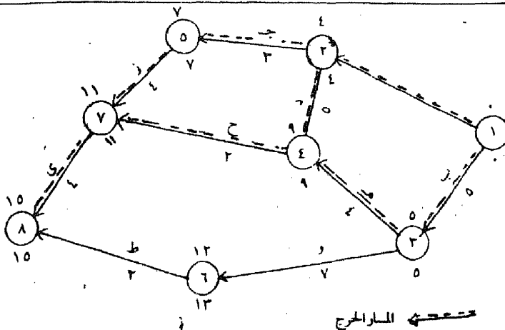
شكل (١٤/٦) تعجيل (أ) أسبوعين
