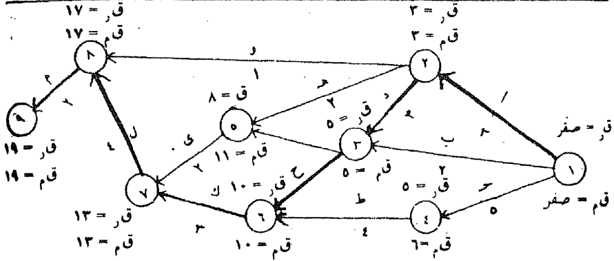
شكل (١/١٥) خريطة التتابع الفني مع ق ر ، ق م للأحداث
