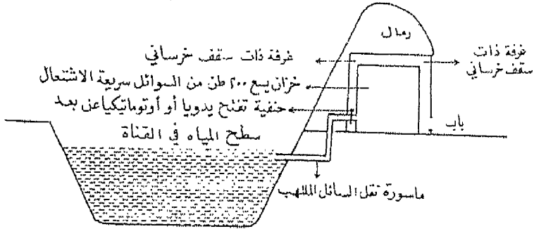
الشكل رقم ٣ رسم تخطيطي يبين أسلوب العدو في إشعال النيران على سطح المياه
